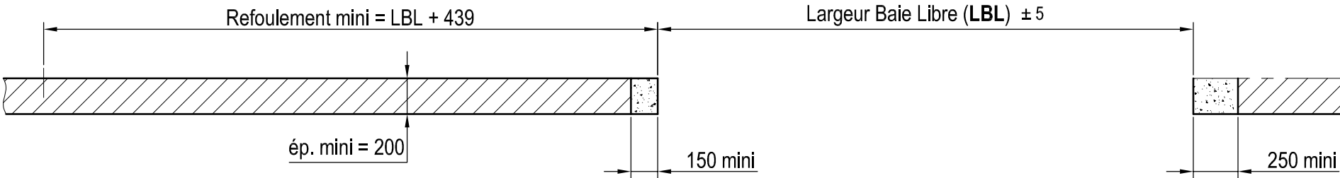
PLAN DE PRINCIPE PORTE COULISSANTE 1 VANTAIL RAIL SOUS DALLE MONTAGE SUR LINTEAU
