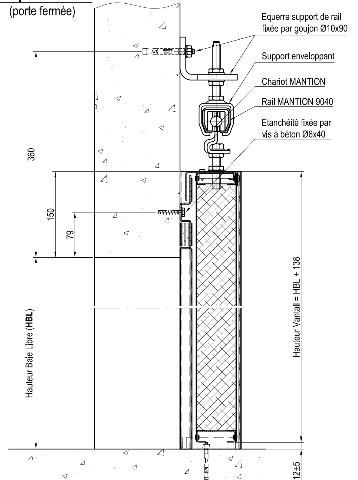
Coupe Verticale
