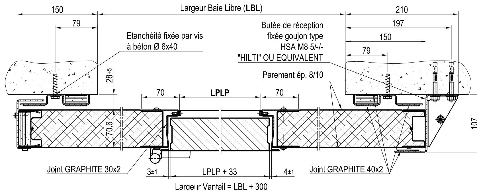
Coupe Horizontale (porte fermée)
