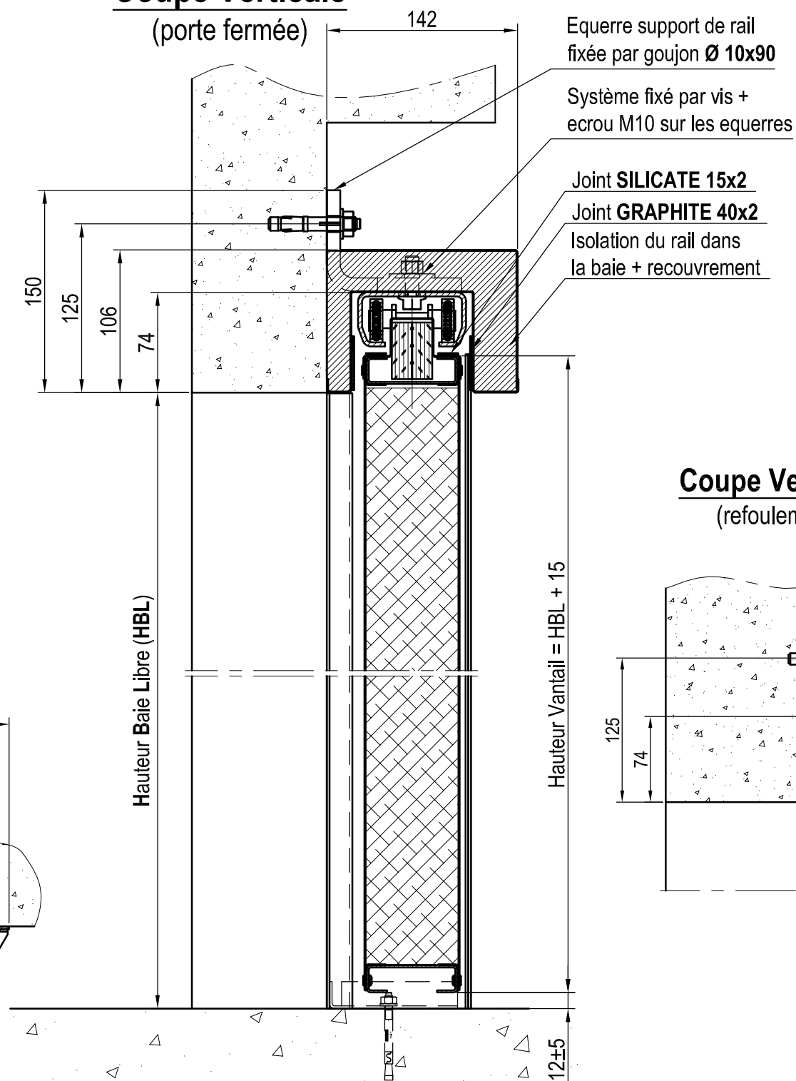
Coupe Verticale
