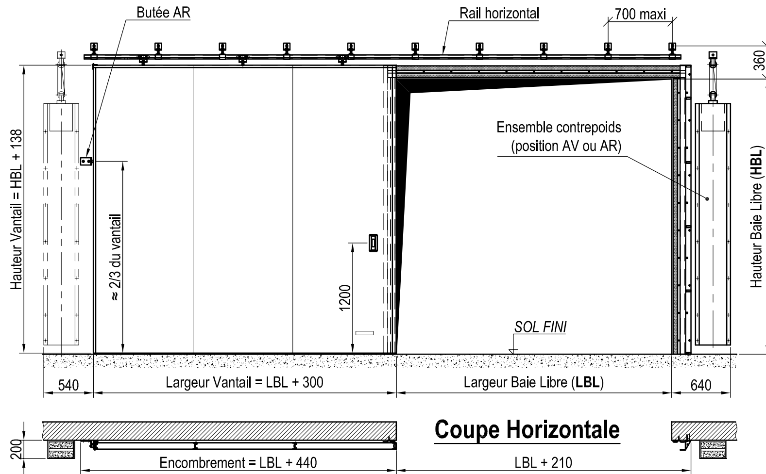
Coupe Horizontale (porte fermée)
