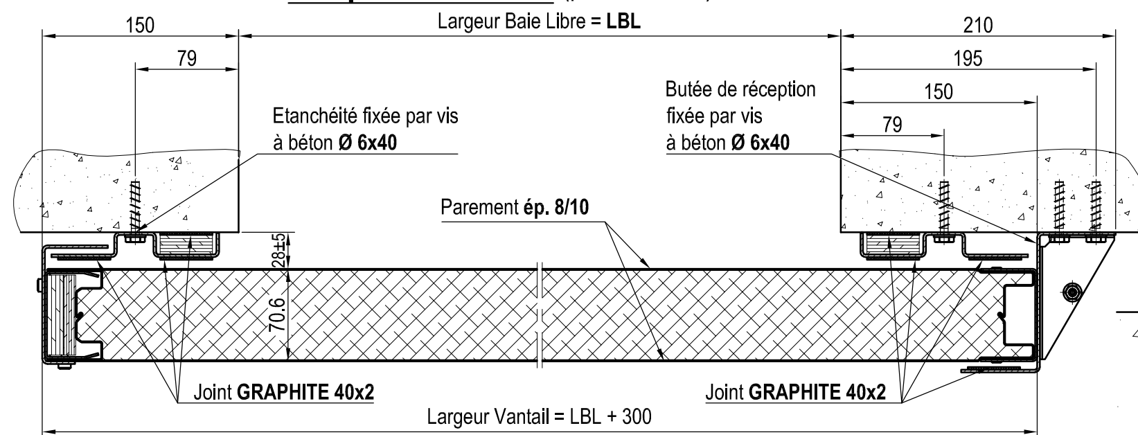
Coupe Horizontale (porte fermée)
